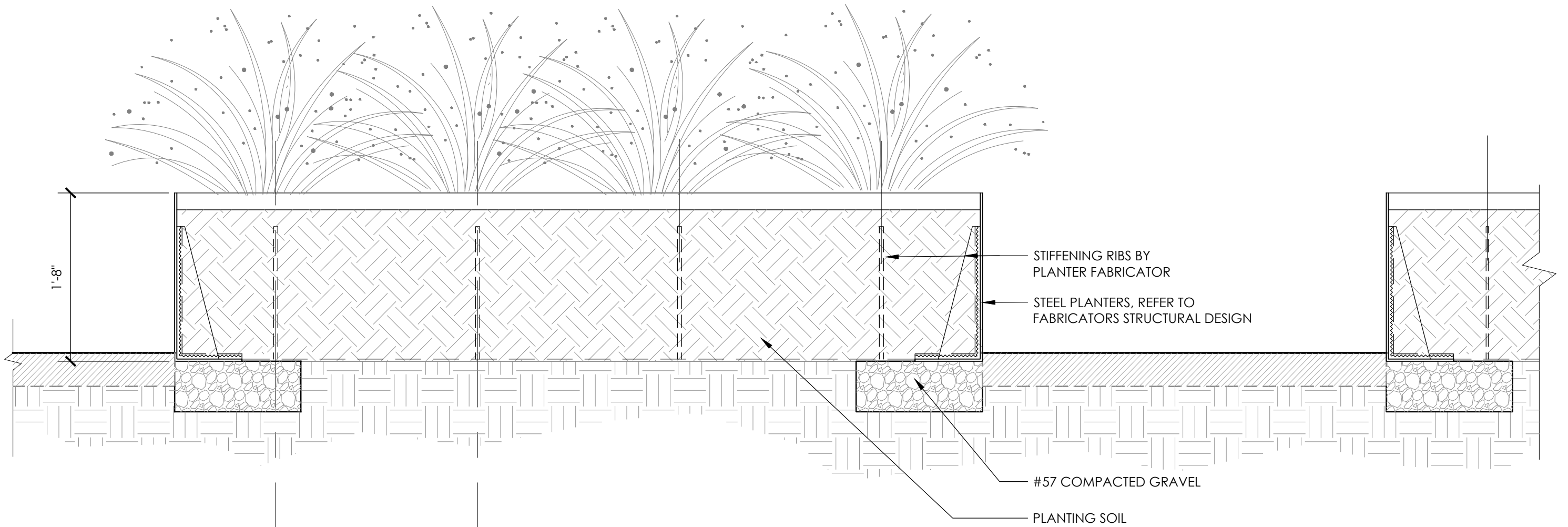
2 ELEVATION SCALE: 1/2"=1'-0"
