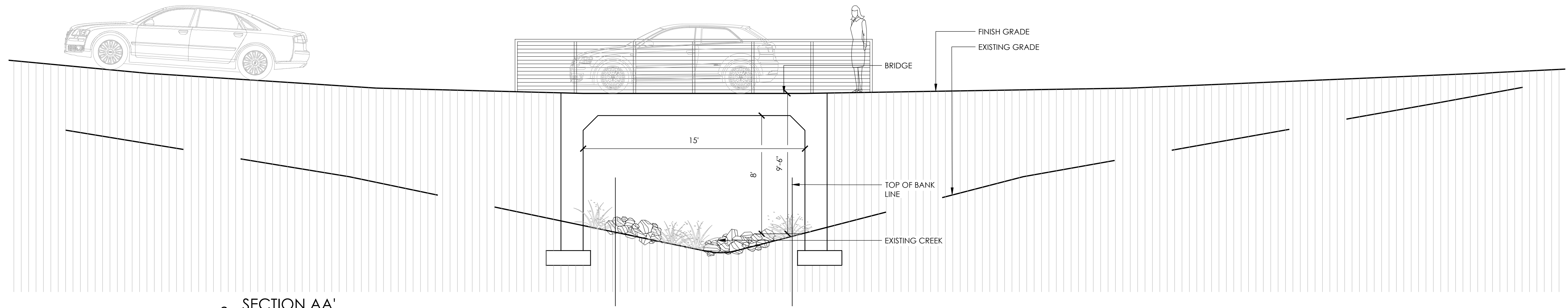
2 SECTION AA' SCALE: 1/4" = 1'-0"
